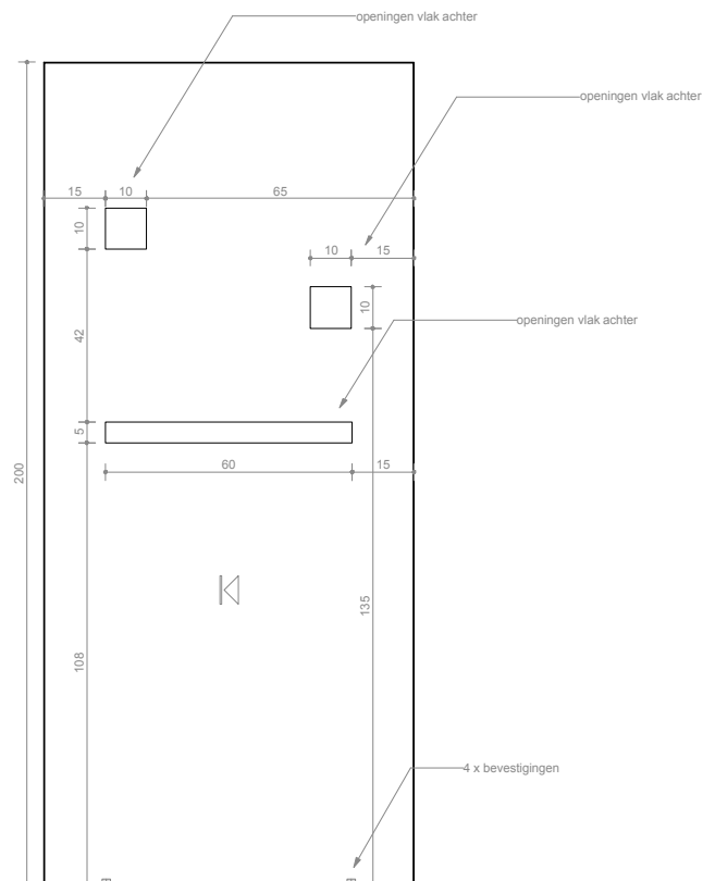
SNEDE - BOVEN
