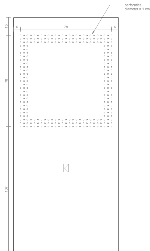
AANZICHT - BOVEN
