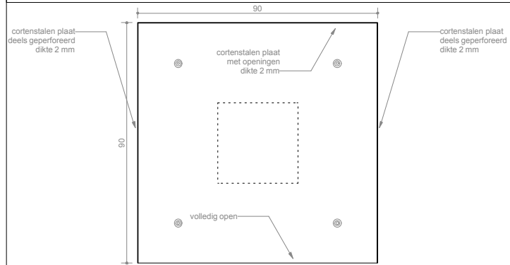
SNEDE - BOVEN
